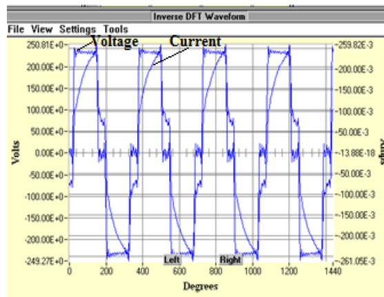
(d) Maximum voltage angle at 133^{\circ}
